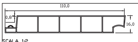
SCALA 1:2 38PE42
