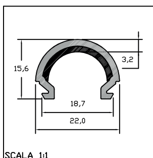
SCALA 1:1 41PE06
