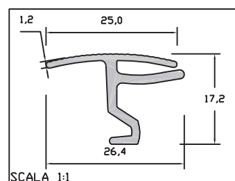
SCALA 1:1 12PE14
