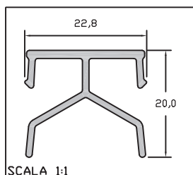
SCALA 1:1 36PE14
