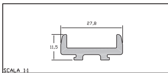
SCALA 1:1 16PE09
