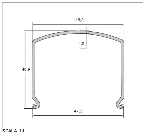
SCALA 1:1 41PE96
