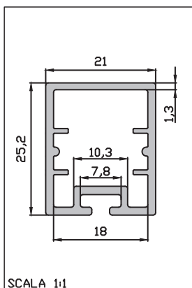
SCALA 1:1 32PE01
