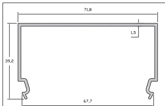
SCALA 1:1 41PE07
