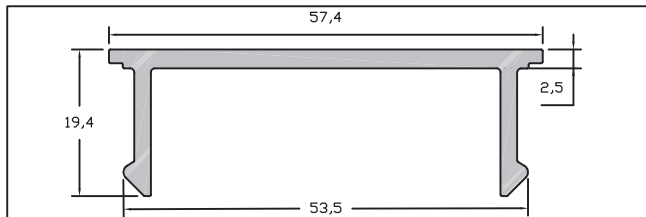
SCALA 1:1 41PE37
