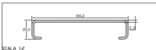
SCALA 1:2 22AE02
