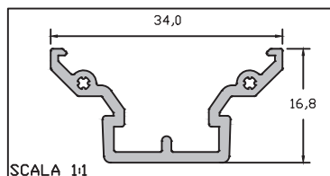
SCALA 1:1 37PE08
